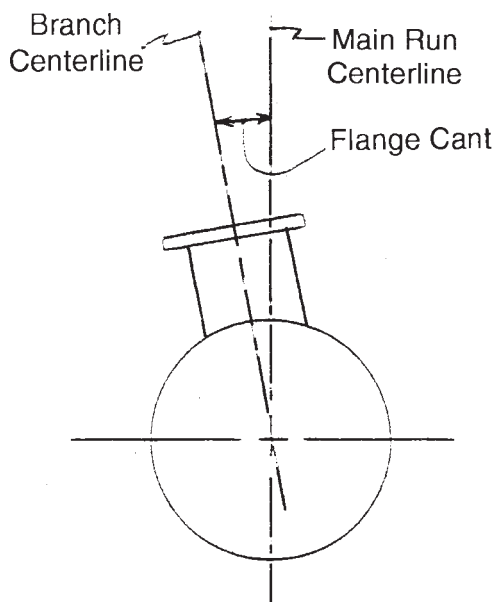
FIG. 1 Flange Cant
