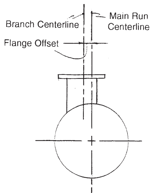
FIG. 3 Flange Offset
